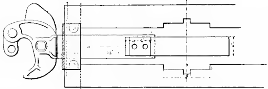
Fig. 2201. Plan.
